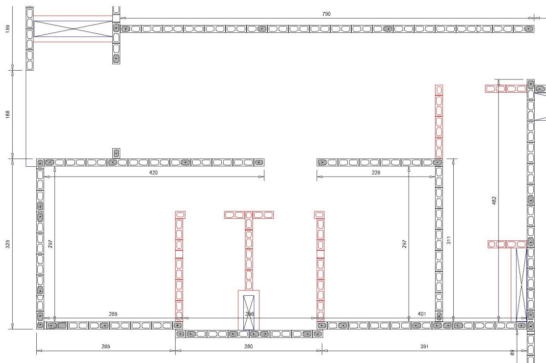
PLANTA PAV. TIPO FINAL 03 S/ ESCALA
