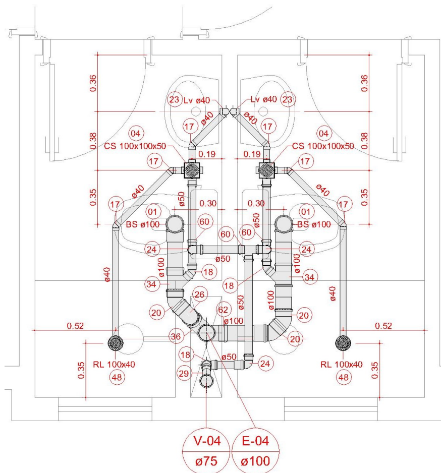
DETALHE ESGOTO BANHEIRO PAV. TIPO FINAL 03 S/ ESCALA
