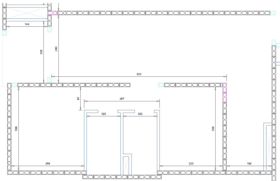
PLANTA PAV. TIPO FINAL 03 – 2ª. FIADA S/ ESCALA
