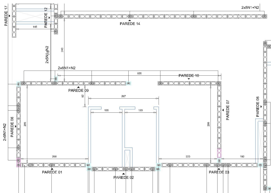
PLANTA PAV. TIPO FINAL 03 – 1ª. FIADA S/ ESCALA
