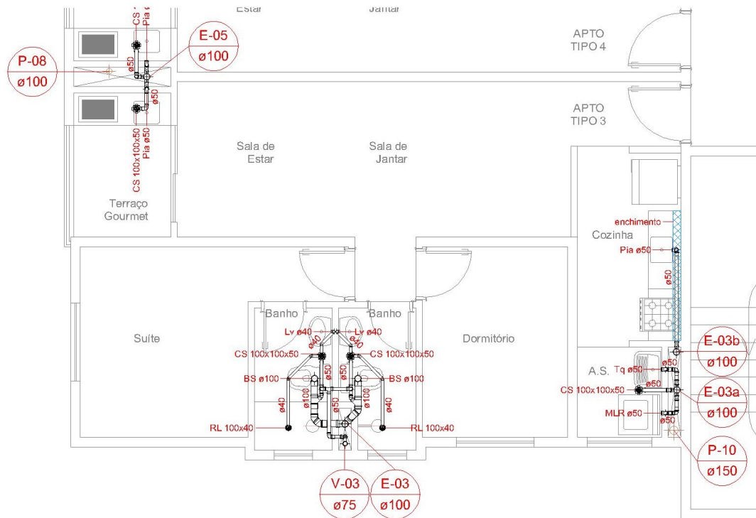
PLANTA PAV. TIPO FINAL 03 S/ ESCALA
