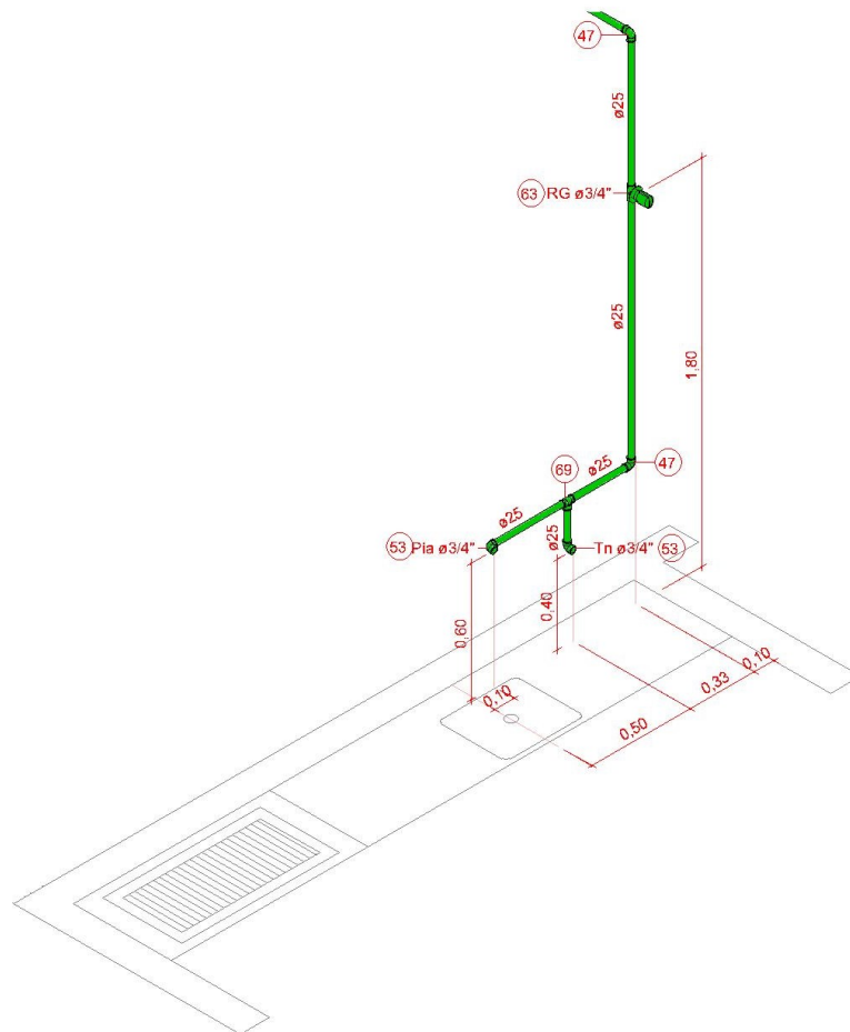
ISOMÉTRICA TERRAÇO – ÁGUA FRIA – FINAL 03 S/ESCALA
