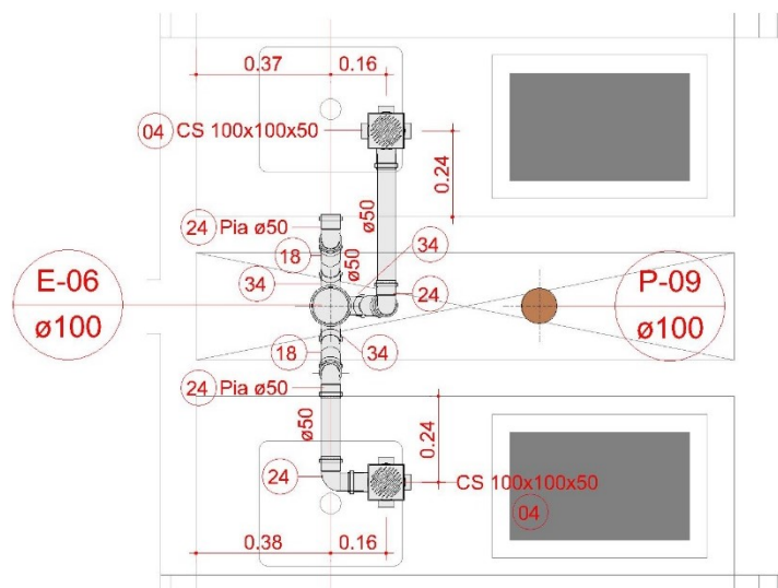
DETALHE ESGOTO TERRAÇO PAV. TIPO FINAL 03 S/ ESCALA
