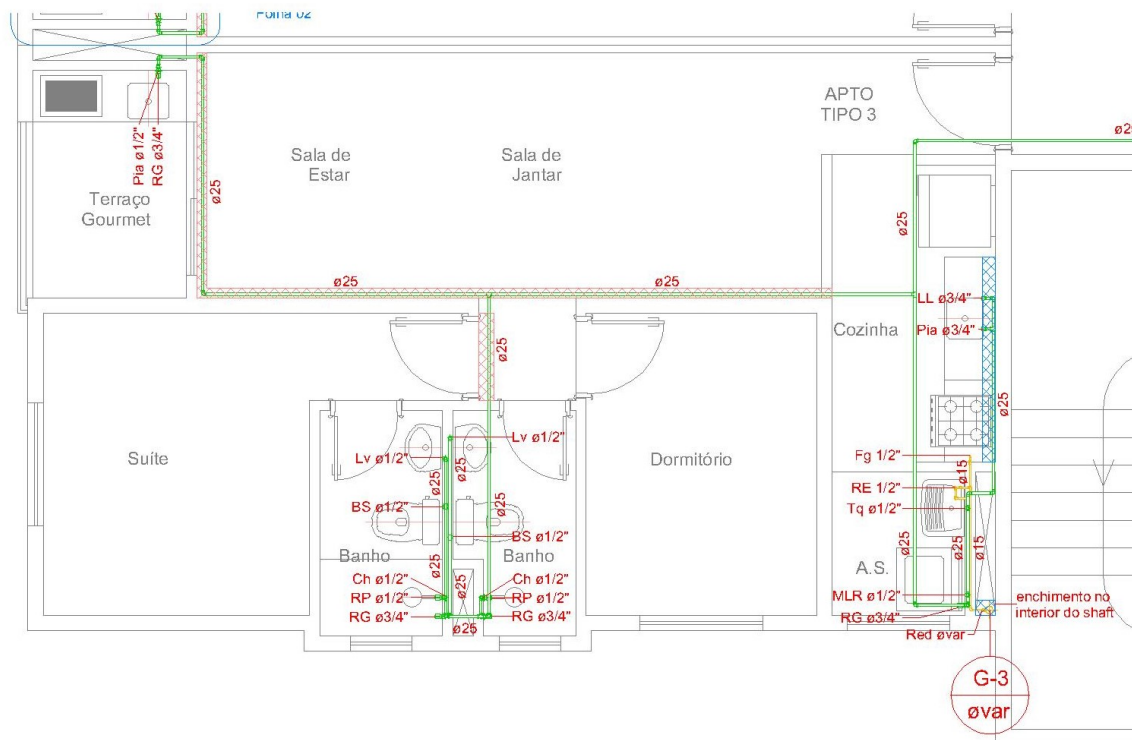
PLANTA PAV. TIPO FINAL 03 S/ ESCALA
