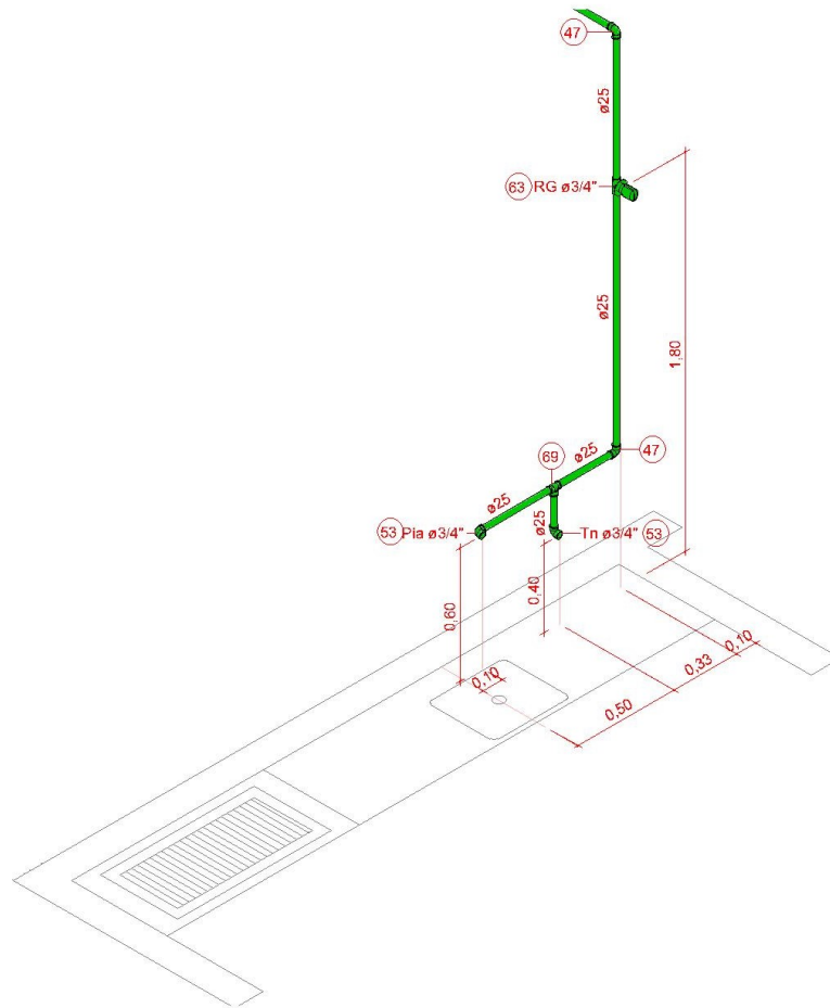
ISOMÉTRICA TERRAÇO – ÁGUA FRIA – FINAL 04 S/ESCALA
