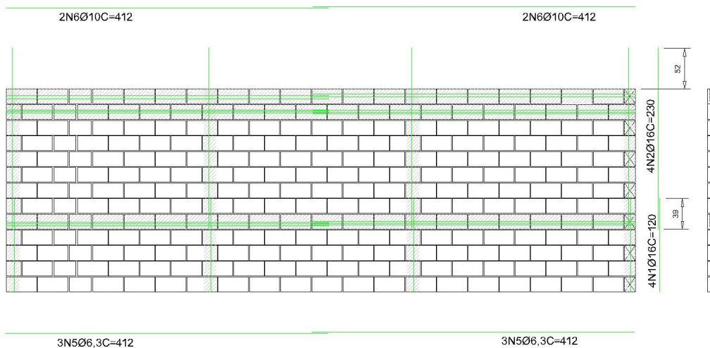
ELEVAÇÕES ALVENARIA ESTRUTURAL S/ ESCALA
