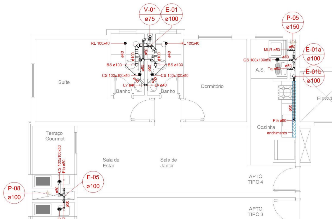
PLANTA PAV. TIPO FINAL 04 S/ ESCALA
