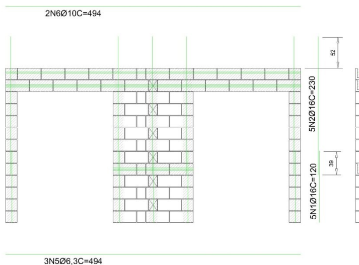
ELEVAÇÕES ALVENARIA ESTRUTURAL S/ ESCALA
