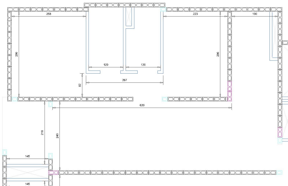
PLANTA PAV. TIPO FINAL 04 – 2ª. FIADA S/ ESCALA
