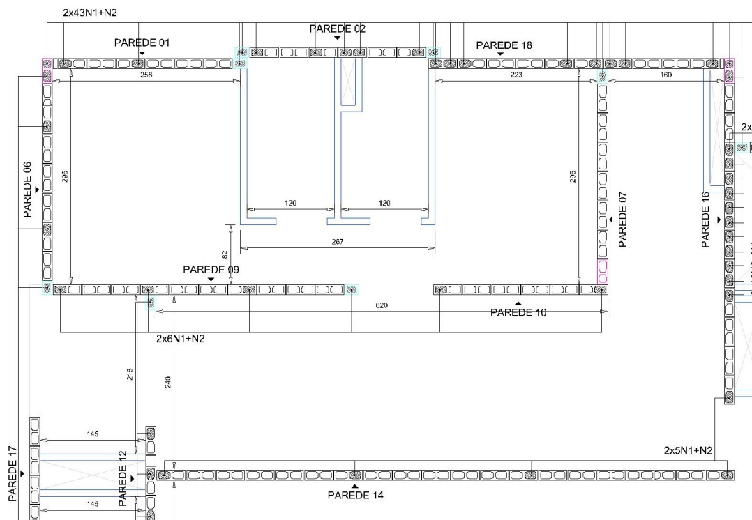
PLANTA PAV. TIPO FINAL 04 – 1ª. FIADA S/ ESCALA
