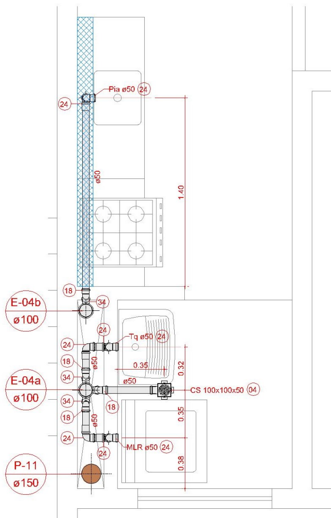
DETALHE ESGOTO COZINHA PAV. TIPO FINAL 04 S/ ESCALA
